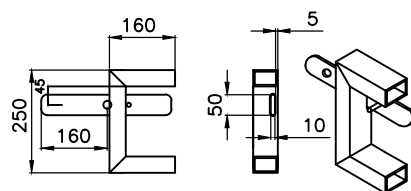
SHOOTBOLT DETAILS
