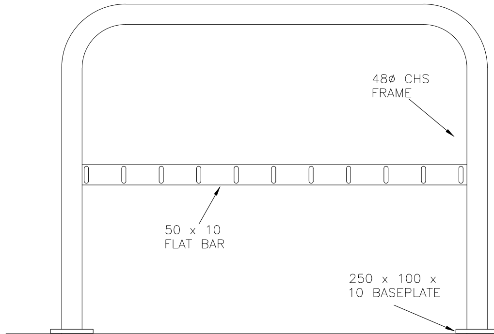
ELEVATION
