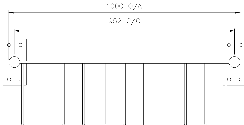
ELEVATION
