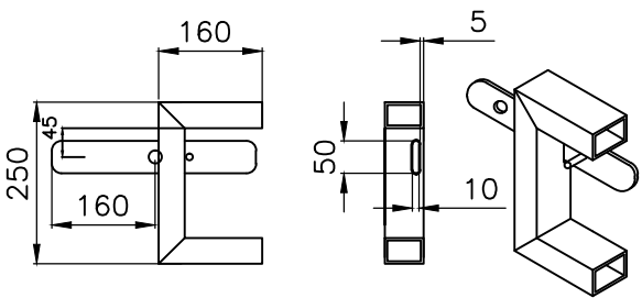
SHOOTBOLT DETAILS
